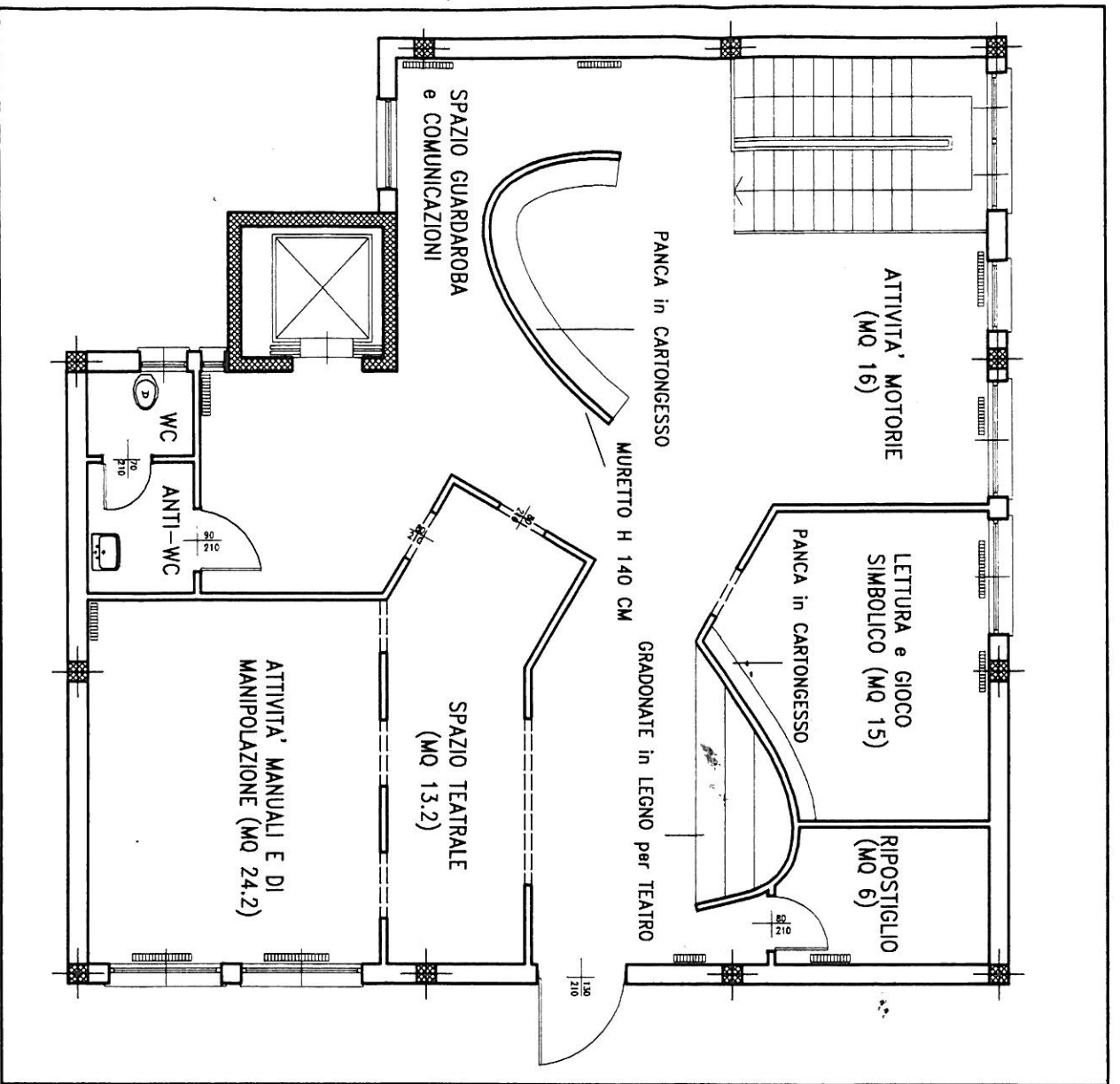
Pianta - Scala 1:100
